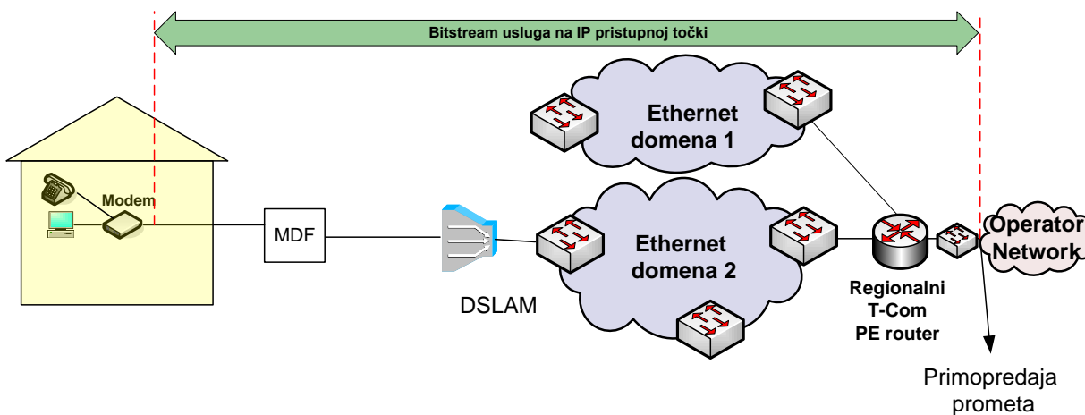
Slika 17. Veleprodajni širokopolasni pristup za pružanje VoIP usluge na IP razini u slučaju kada Krajnji korisnik ostvaruje Osnovni pristup mreži putem usluge Operatora korisnika
